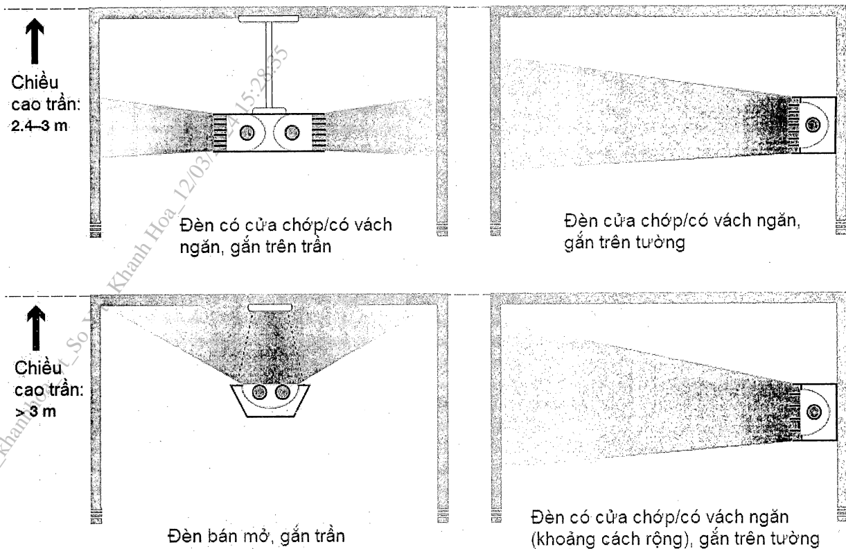
Hình 8: Các loại đèn GUV tầng trên phù hợp với chiều cao phòng khác nhau 20
